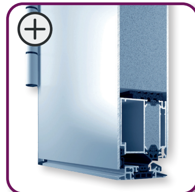
Innenansicht Aufsatzfüllung beidseitig [Ud-Wert \leq 1,0 \text{ /m}^2\text{K} ]
