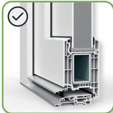
Außenansicht Einsatzfüllung [Ud-Wert \leq 1,2 / m^2K ]
