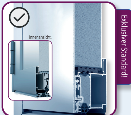
Außenansicht Aufsatzfüllung einseitig [Ud-Wert \leq 1,2 \text{ /m}^2\text{K} ]
