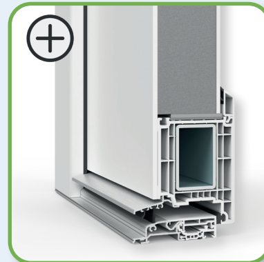
Außenansicht Aufsatzfüllung einseitig [Ud-Wert \leq 1,0 / m^2K ]
